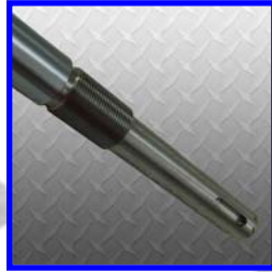
AS-EM120-01-00-37 Arbor/Shaft
